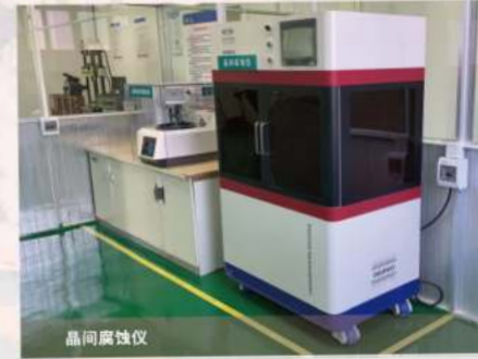
晶间腐蚀仪
